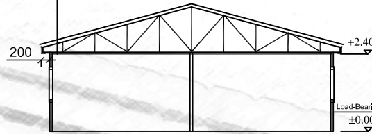
A-A SECTION
