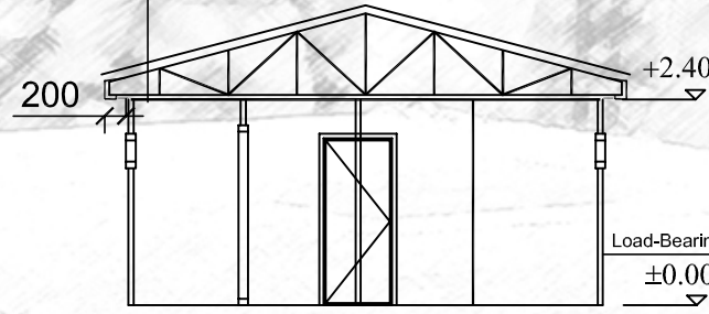
A-A SECTION
