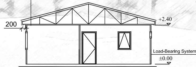
A-A SECTION
