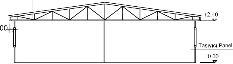
A-A KESİTİ
