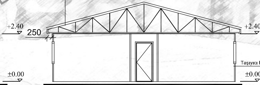
A-A KESİTİ
