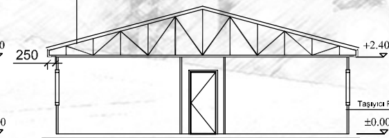
A-A KESİTİ
