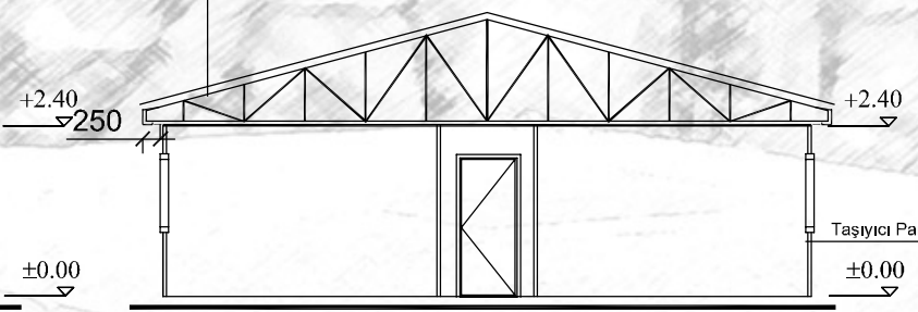
A-A KESİTİ
