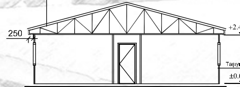
A-A KESİTİ
