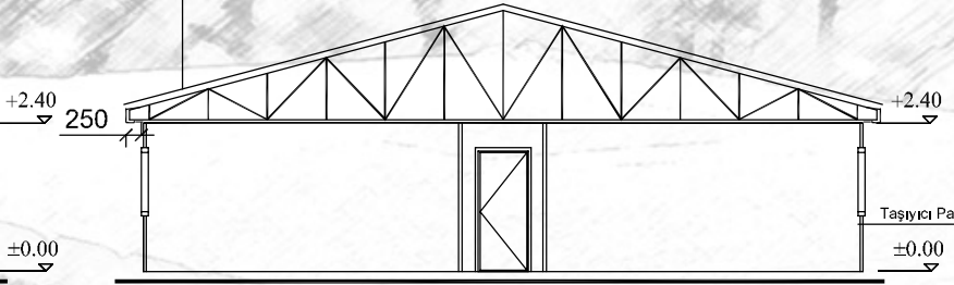
A-A KESİTİ
