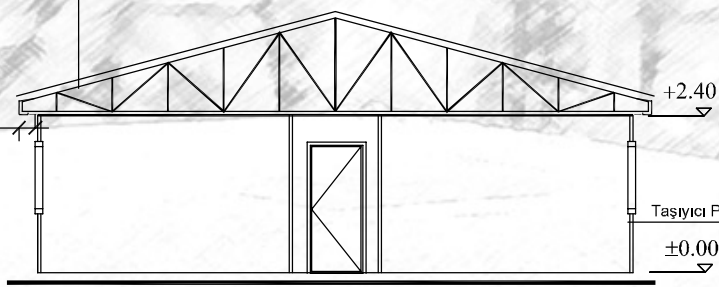
A-A KESİTİ
