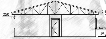
A-A KESİTİ
